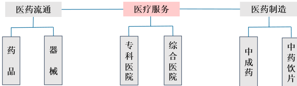
业务架构
