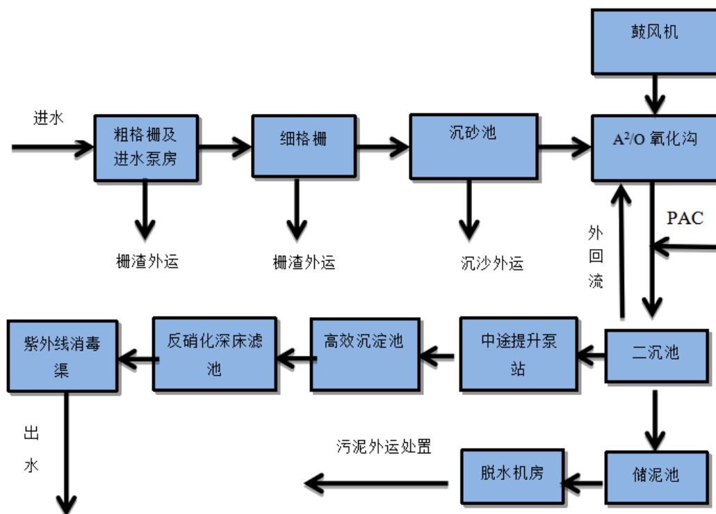
图：发行人污水处理工艺流程图
